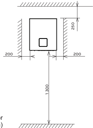
Minimální servisní prostor (jednotka: mm)
